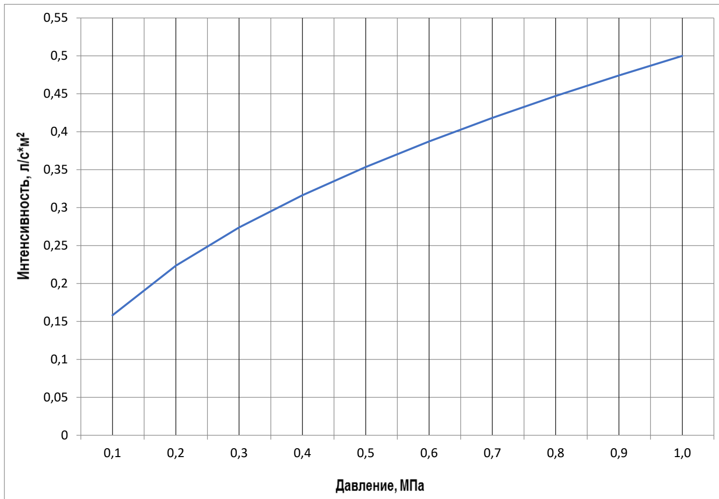
График зависимости интенсивности орошения от давления на площади 12 м 2 , защищаемой группой оросителей (два и более) с высоты 2,5 м
